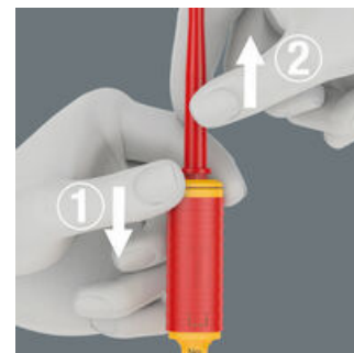
Pociągnięcie w dół i przytrzymanie przycisku zwalniającego powoduje zwolnienie blokady. Trzpień wymienny lub klucz do szaf sterowniczych może zostać usunięty.
