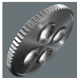
Den fintannede mekanismen med 60 tenner gir en returvinkel på kun 6° - ideelt for presisjonsarbeid.
