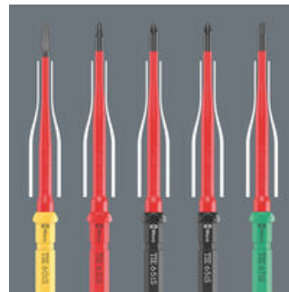
Redusert klingediameter med integrert beskyttelsesisolering som gir enkel tilgang til dyptsittende skruer og fjærelementer, testet enkeltvis i henhold til IEC 60900.
