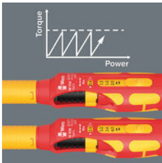
Dreiemomentfunksjon med utløsningsmekanisme for tiltrekking mot høyre/venstre forhindrer utilsiktet overføring av for høye dreiemomenter.
