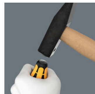
De schroefbeitel met geïntegreerde slagkap
