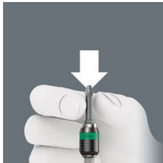
커버를 그대로 두고 비트를 어댑터 안으로 밀어넣을 수 있음. 비트가 나사에 고정되는 잠금 장치가 자동으로 활성화되어 흔들림 없이 안전하게 고정됨.
