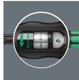
トルク値の設定および保存が簡単にできます。メインスケールとファインスケールで目盛りが読みやすくなっています。
