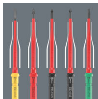
電気工事用 差替式絶縁ブレード、スリム軸
