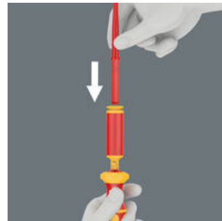
La lame interchangeable, munie du profil de sortie requis ou d'une clé pour armoire électrique en fonction de ce qu'exige la tâche, se glisse dans le logement du manche.
