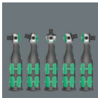
La tête du cliquet est librement orientable et peut être déverrouillée en toute position grâce au bouton coulissant positionné sur les 2 côtés. Travail sans problème et avec une grande liberté de manœuvre, même dans les endroits très exigus ou difficiles d'accès. Les positions de blocage définies à 0°, 15° et 90° à gauche et à droite garantissent un travail sûr et empêchent la tête de ripper.
