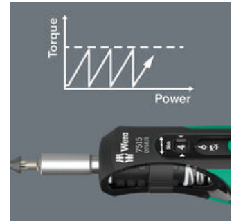
Se oye y se palpa claramente el sobre-encastre tan pronto se alcanza el par de apriete preajustado.
