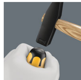
Skrueværktøjsæt er udstyret med en integreret slagkappe til forøgelse af levetiden og reduktion af splintringsrisikoen. Alligevel gælder principielt: Brug beskyttelsesbriller!
