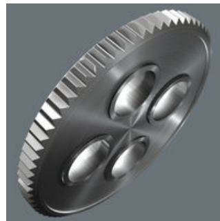
Jemná zubová mechanika se 60 zuby umožňuje malý úhel zpětného otočení 6° pro přesnou práci.
