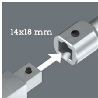
Prodlužovací páka 9999 je vhodný pro nástrčné nástroje se čtyřhranným pohonem 14x18 mm. Díky tomu lze nástroj použít pro širokou škálu aplikací.
