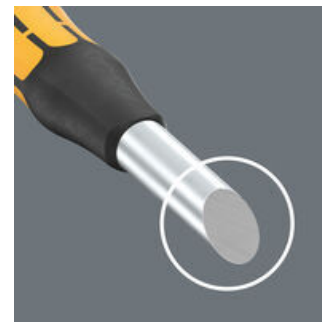
Matný chromovaný plný materiál ze speciální legované oceli nabízí vysokou rozměrovou stabilitu a díky zvýšené pevnosti je odolný proti deformacím.
