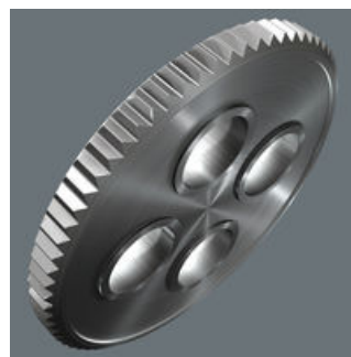
棘轮采用60齿细齿结构, 6°回转角是精密作业的理想选择。
