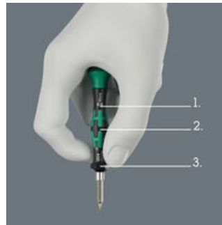
Kraftform Micro 1014 批头夹持螺丝刀
