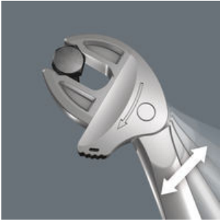
Joker 6004: 快速工作的棘轮机构
