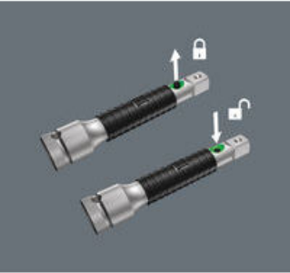
活锁装置
